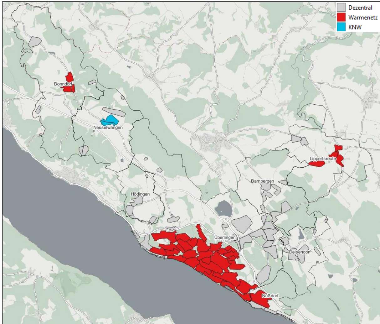
Abbildung 30: Zielfoto 2040 Versorgungssysteme der Cluster
