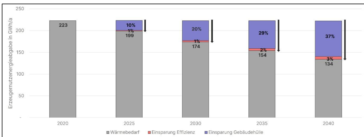
Abbildung 9: Energiebedarfsentwicklung – Szenario 1
