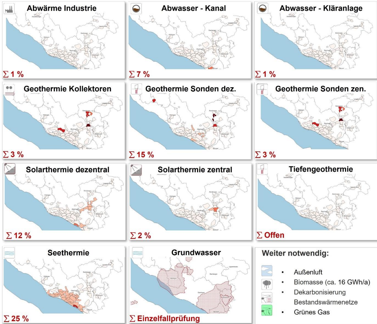
Abbildung 27: Übersicht der Einzelpotenziale zur Bedarfsdeckung im Bereich Wärme
