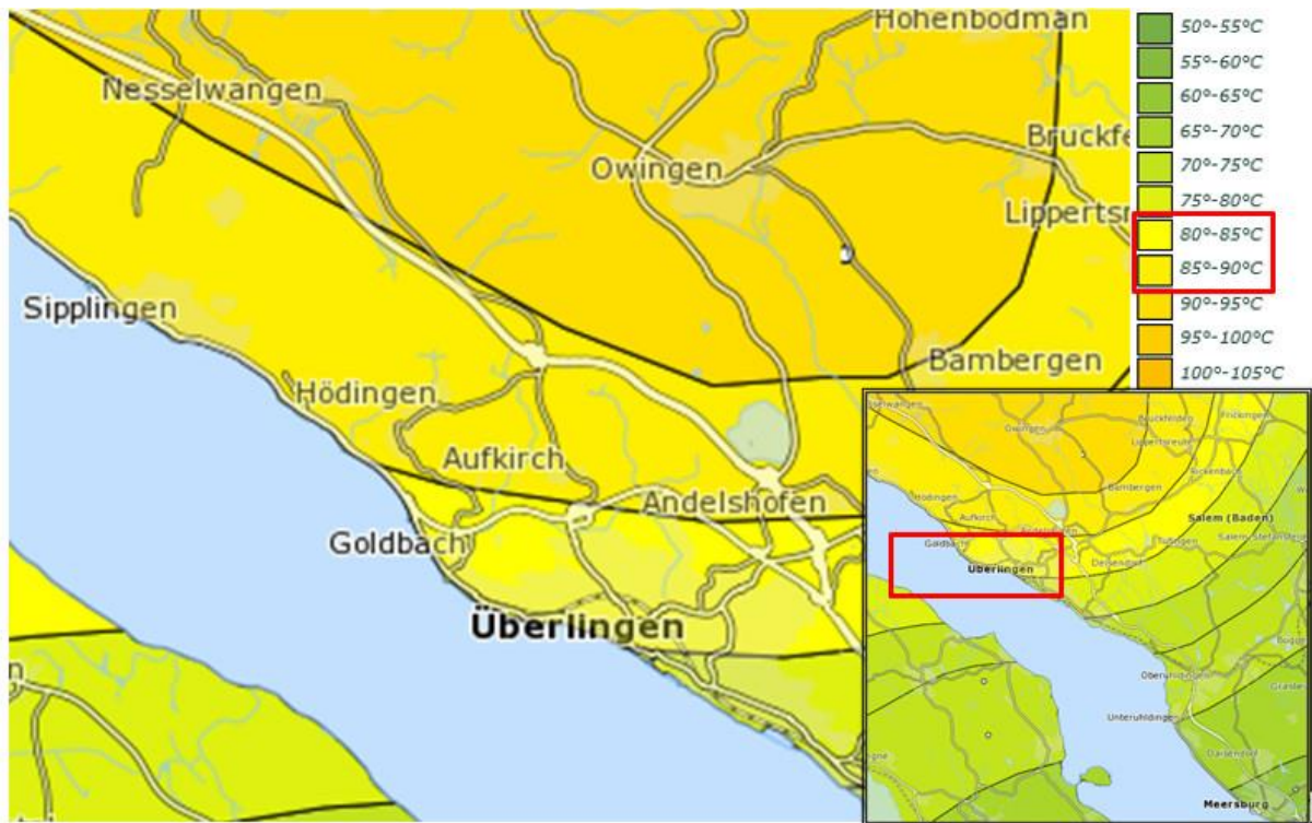
Abbildung 21: Potenzialkarte „Tiefengeothermie“ in 1.500 m
