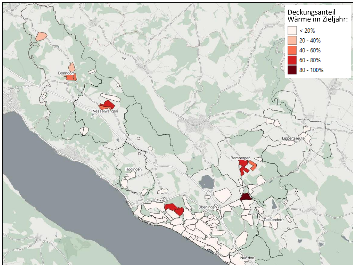
Abbildung 12: Potenzialkarte „Geothermie – Kollektoren zentral“ auf Clusterebene
