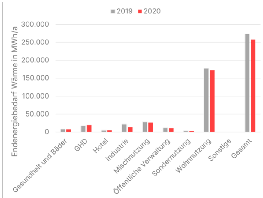
Abbildung 6: Endenergiebedarf Wärme nach Nutzungssektoren
