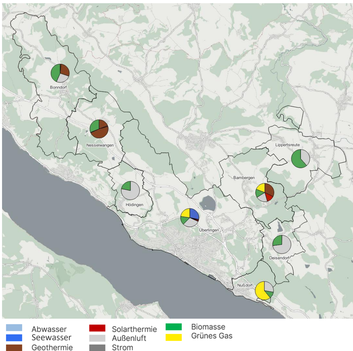
Abbildung 29: Zielfoto 2040 Energieversorgung der Stadtteile
