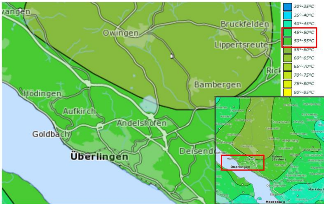
Abbildung 40: Temperatur in 1.000 m Tiefe
