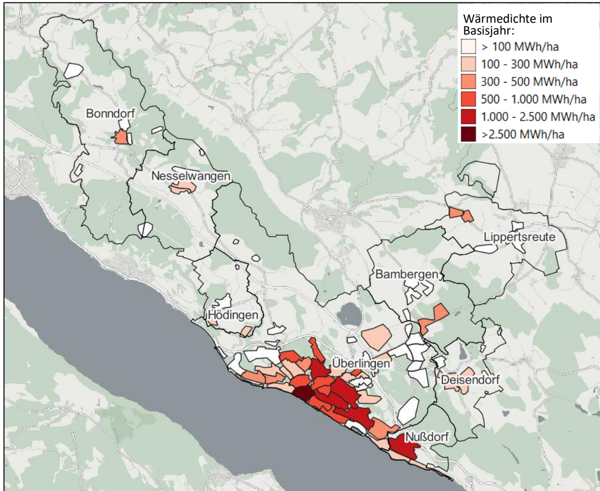
Abbildung 5: Wärmedichte je Cluster
