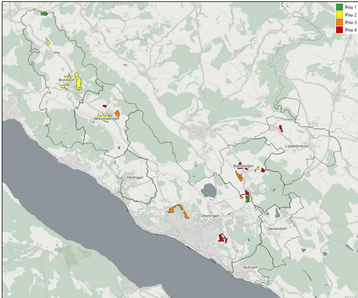
Abbildung 24: Potenzialkarte Freiflächen „Photovoltaik – zentral“
