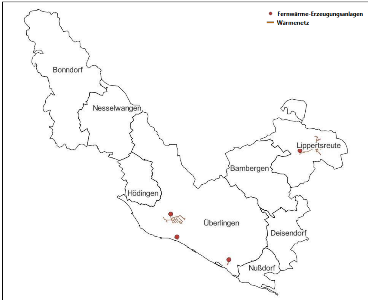
Abbildung 3: Übersichtskarte der Wärmenetze
