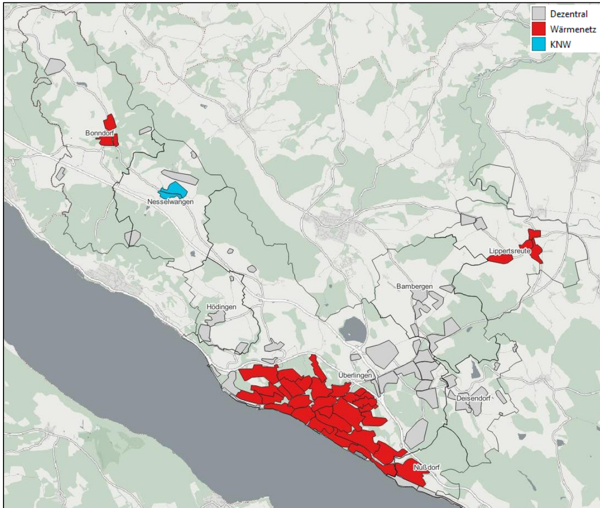
Abbildung 32: Clusterkarte mit Wärmenetzgebieten aus dem Zielfoto 2040
